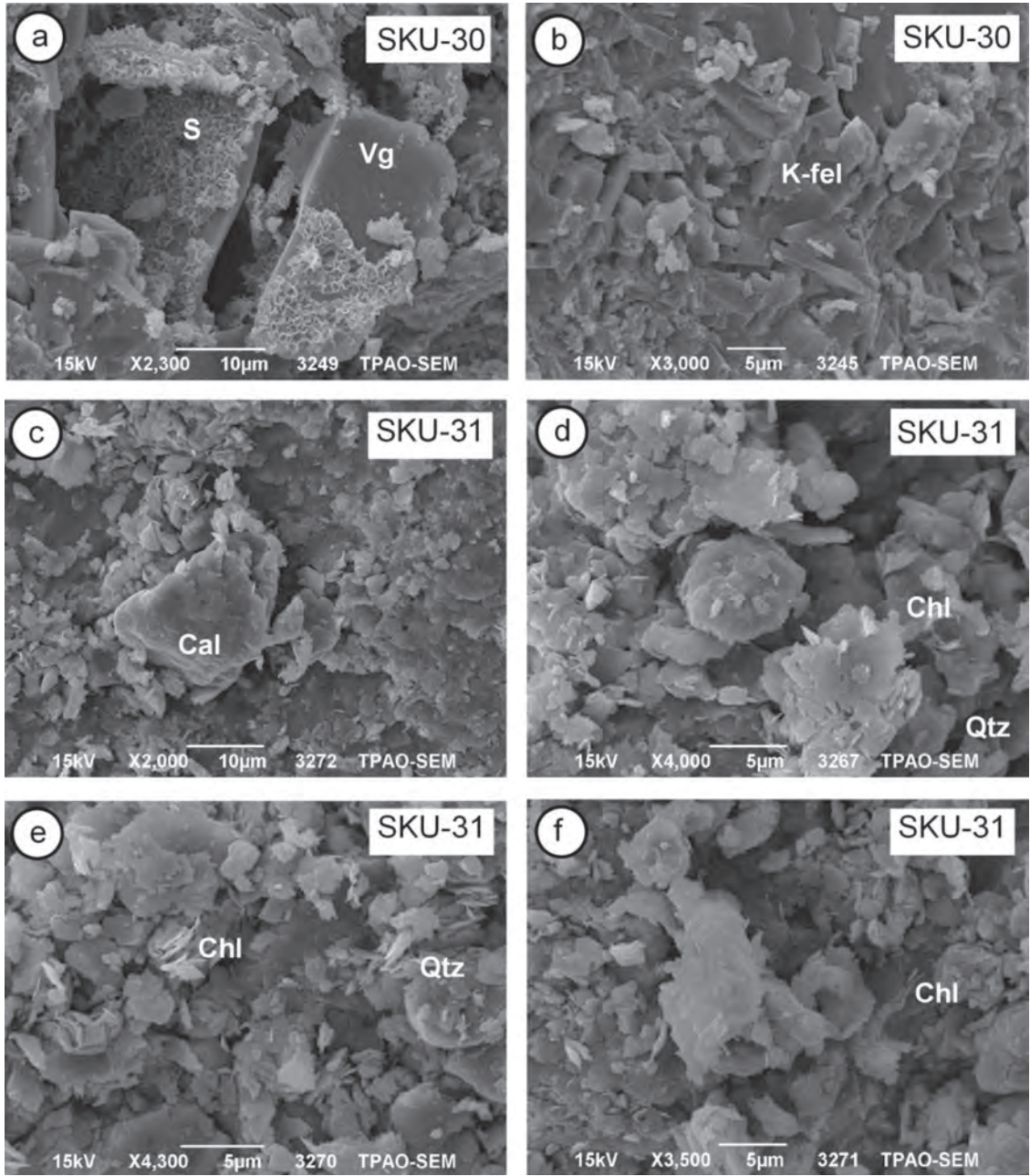
Şekil 6. Yapalı Üyesi örneklerinin SEM mikrofotografaları (Vg=Volkanik camı, S=Smektit, K-fel=K-feldispat, Cal=Kalsit, C-S=Karışık tabakalı klorit-smektit, Chl=Klorit, Qtz=Kuvars), tüflü silttaşı: a) Volkanik camdan itibaren gelişmiş bal-peteği dokulu smektitler, b) Levhamsı prizmatik K-feldispatlar; şeyl: c) Özşekilsiz kalsit mineralleri, d) Yapraksı klorit mineralleri, e) Kloritik matriks içerisinde özşekilli kuvars, f) Kıvrılmış iri klorit yaprakları.
