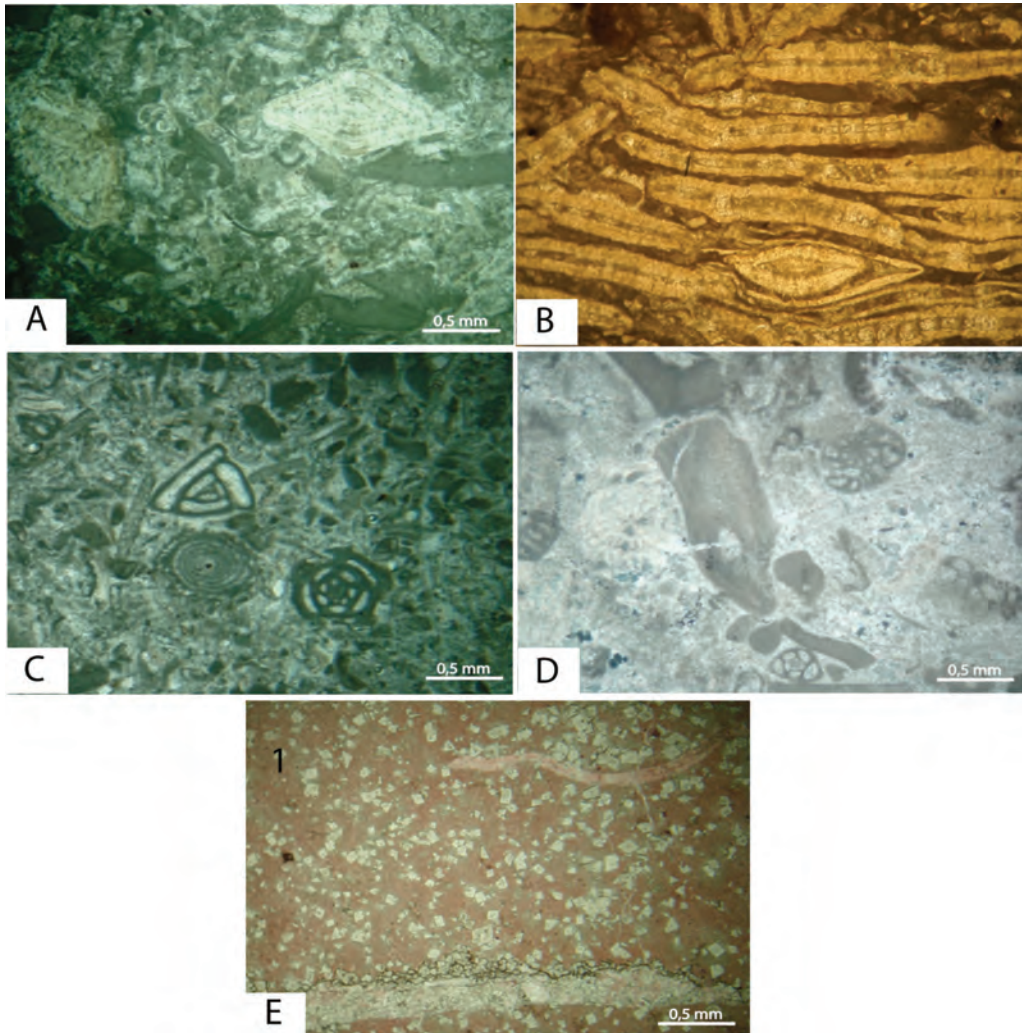
Şekil 6. Resif önu (A- B) ve resif ardı (C- D- E) fasiyesi fotoğrafları: A) büyük bentik foraminiferli- algli istiflaş mikrofasisesi; B) Operculinali istiflaş mikrofasisesi; C) küçük bentik foraminiferli-algli istiflaş mikrofasisesi; D) küçük bentik foraminiferli-algli vaketaşı mikrofasisesi; E) biyoklastlı vaketaşı- çamurtaşı mikrofasisesi. Kesitte ayrıca saçılmış halde geç diyajenetik dolomit kristalleri görülmektedir.
