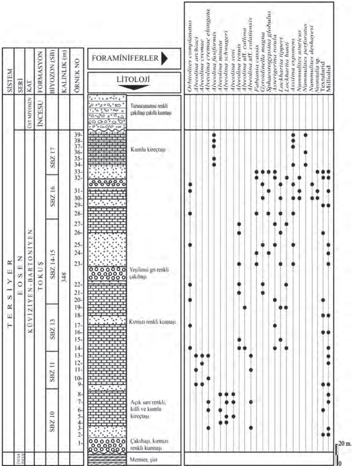
Şekil 3. Alaman ölçülü stratigrafi kesiti Figure 3. Alaman measured stratigraphy section
